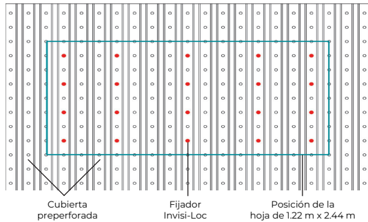
Figura A Patrón de cuadrícula para estructura acanalada para Invisi-Loc®
